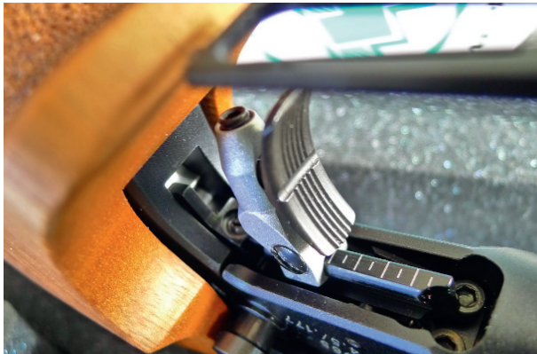
Pistol på rygg, med blottet avtrekksmekanisme. Ikke noe erotisk i dette, bare for å ha det nevnt. Her kan justerskruene, som er lette å komme til, beskes.
