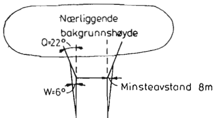
Figur 17 A Farlig område i horisontalplanet
