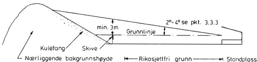
Figur 17 B Terrangsnitt i vertikalplanet
