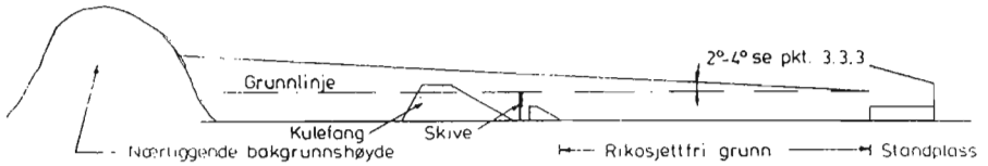
Figur 13B Terrengsnitt i vertikalplanet.
