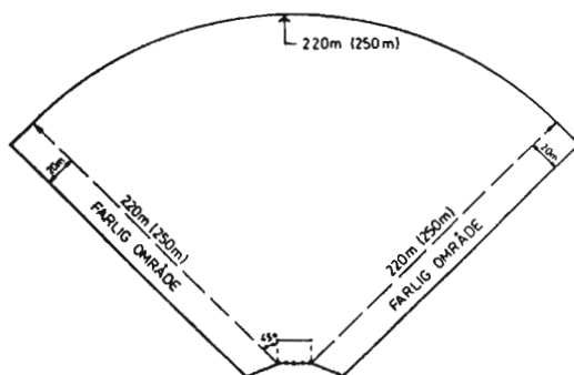
Figur 19 Lerduebane – olympisk trap
