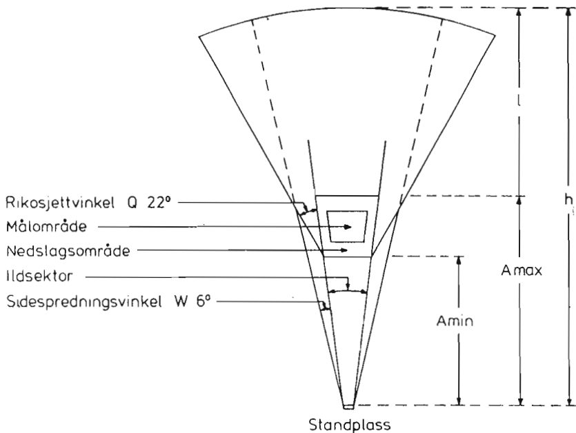
Figur 1 Eksempel på sikkerhetsmal for skytebane
