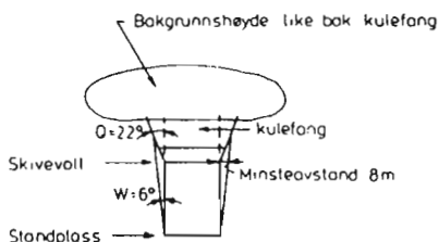
Figur 18 A Farlig område i horisontalplanet
