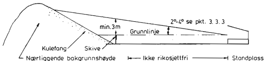
Figur 16 B Terrøngsnitt i vertikalplanet
