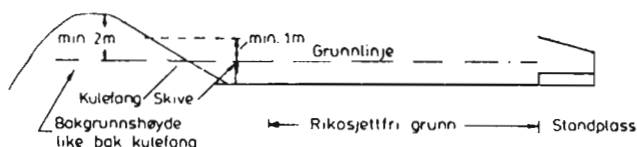
Figur 18 B Terrengsnitt i vertikalplanet
