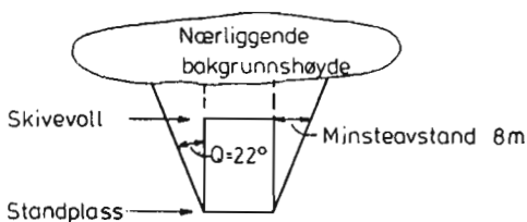
Figur 16 A Farlig område i horisontalplanet
