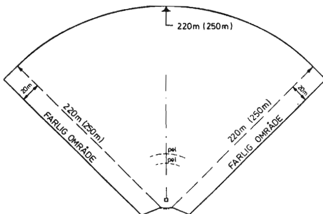
Figur 22 Lerduebane – jegertrap
