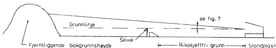
Figur 12B Terrengsnitt i vertikalplanet.
