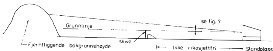
Figur 11B Terrengsnitt i vertikalplanet.
