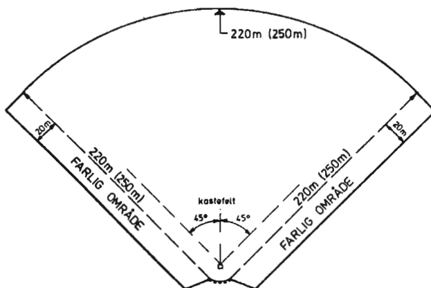
Figur 20 Lerduebane – automatisk trap
