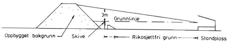
Figur 14B Terrengsnitt i vertikalplanet.
