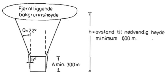
Figur 12A Farlig område i horisontalplanet.
