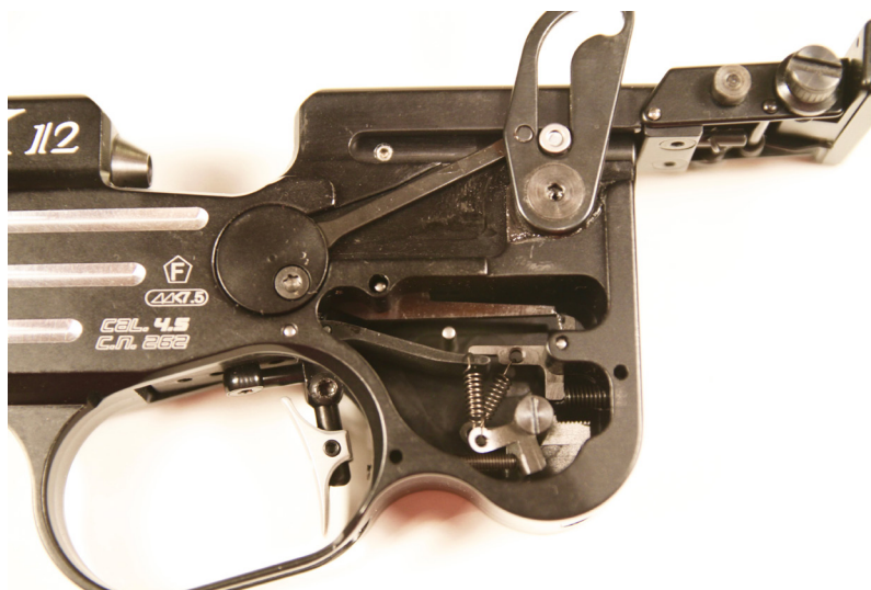
Skjeftet er tatt av, og nå ser man rett inn i avtrekksmekanismen. Dette gjør det enkelt å lære seg hvordan mekanismen fungerer og hvilke skruer man skal skru på for å justere avtrekket slik man vil ha det.
